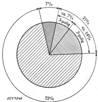
SEV 7540 72% 7% ca. 7% 3-polig 2-polig ca. 14% Kurzschlüsse mit bleibendem Charakter Drei- und zweipolige Lichtbogenkurzschlüsse Erdschlüsse
