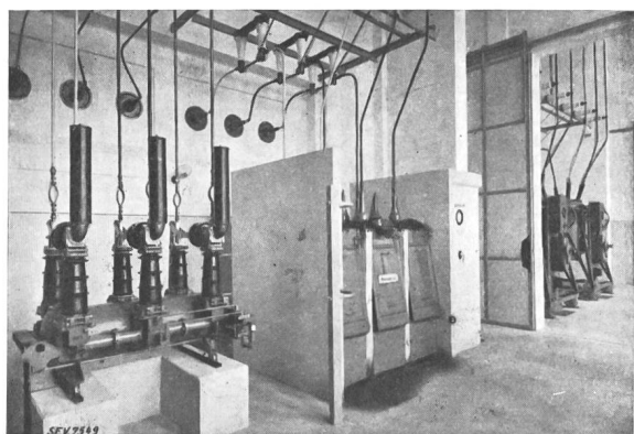
Fig. 42. Ersatz von 50-kV-Oelschaltern durch Druckluftschnellschalter.
