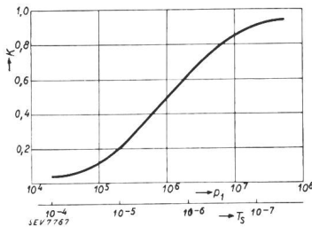
Fig. 17. Berechnete Abhängigkeit der kapazitiv übertragenen Teilspannung von der Steilheit der ankommenden Stoßspannung.
