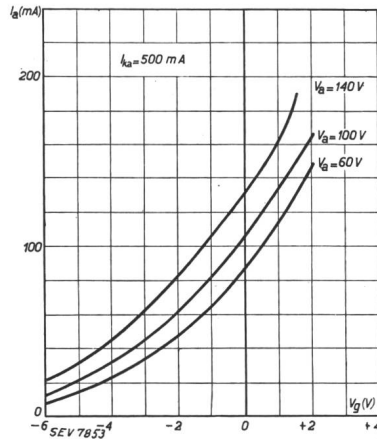
Fig. 4. Kennlinien des Anodenstroms i_a als Funktion der Gitterspannung V_g bei verschiedenen Werten der Anodenspannung V_a . Der Kathodenstrom i_{ka} ist 500 mA.
