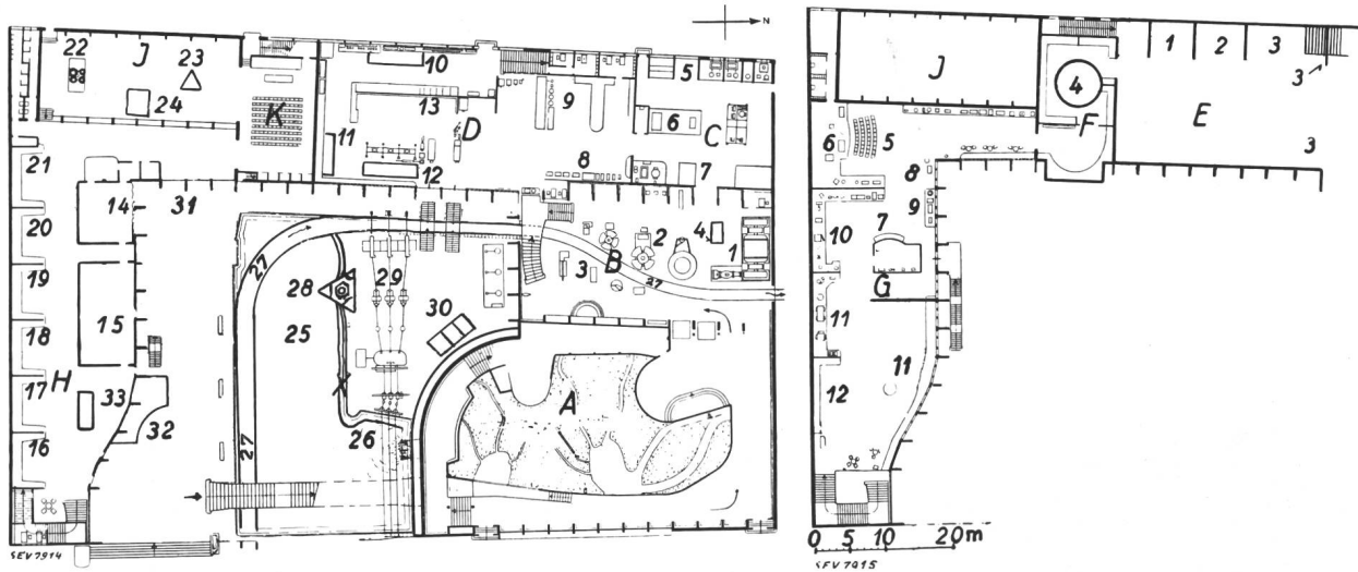
Fig. 2. Grundriss der Abteilung Elektrizität.
