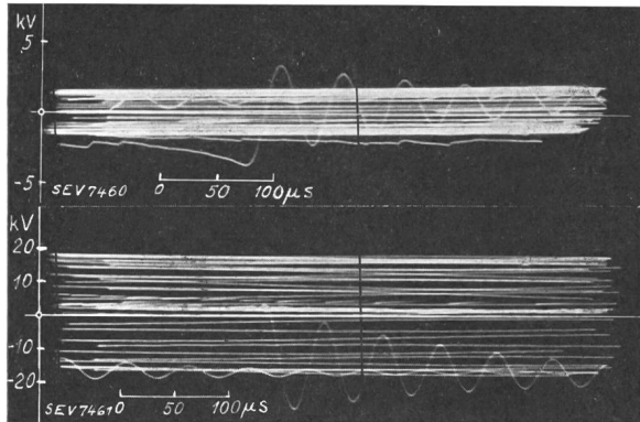
Fig. 6. Einwirkung der Lichtbogenlöscheinrichtung auf die wiederkehrende Spannung.
