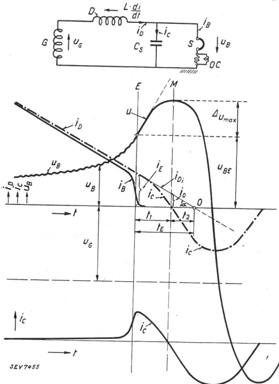
Fig. 1 (oben). Ersatzschema eines Kurzschlusskreises. Fig. 2 (unten). Verlauf von Strom und Spannung bei der Abschaltung eines Wechselstromlichtbogens.
