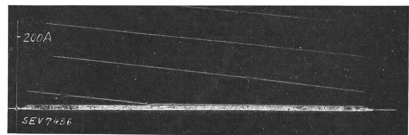
Fig. 3. Kathodenoszillogramm eines Wechselstromes.
