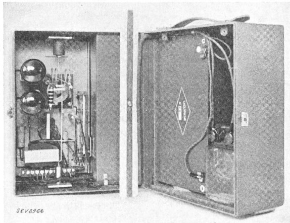
Fig. 2. Kombinierter Sender/Empfänger.
