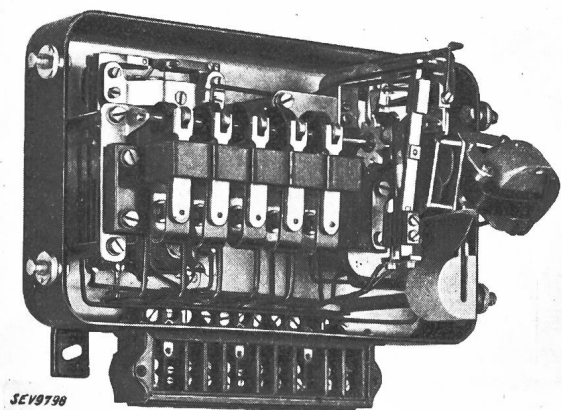
Fig. 2. Blindlast-Regelanlage: Stufenschalter.
