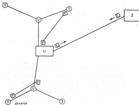
Fig. 12. Schematische Darstellung der Verwendung von UKW-Patrouillengeräten für Störpatrouillen längs Hochspannungsleitungen.
