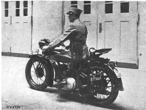
Fig. 11. Polizei-Motorradfahrer mit tragbarem Empfänger.
