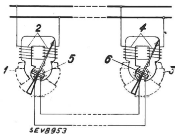
Fig. 1. Grundhaltung der Fernmessung. 1 und 3: Geber bzw. Empf. 2 und 4: deren Feldwicklg. 5 und 6: deren Drehspulen.
