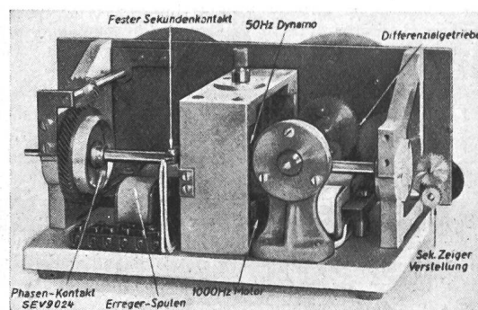
Fig. 5. Rückseite der Synchronuhr mit Differentialgetriebe und Phasenkontakt.
