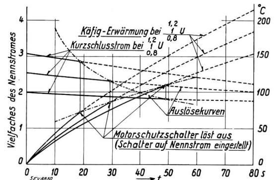
Fig. 14. Erwärmungskurven der Käfigwicklung bei Drehstromspeisung des Stators und festgebremstem Rotor. Drehstrom Combi-Motor Typ 51c, 4polig, 5,5 kW, 380 V, 11,7 A, 50 Hz, 1420 U/min.
