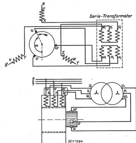
Fig. 7. Drehstrom-Serie-Kommutatormotor (Prinzipschema).
