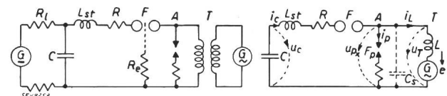
Fig. 4a. Prinzipschema für die Löschkprüfung von Ueberspannungsableitern.
