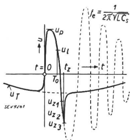
Fig. 6. Spannungsverlauf beim Ansprechen eines Ableiters im Prüfkreis nach Fig. 4. u_T Spannung am Transformator T u_p Restspannung am Ableiter A nach dem Ansprechen im Moment t=0 . u_l Löschspannung am Ableiter im Zeitpunkt t=T_0 . u_{z1}, u_{z2}, u_{z3} Spannungswerte von Rückzündungen im Zeitpunkt t=t_z .
