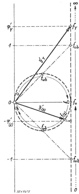
Fig. 4. Reduziertes Vektordiagramm für Serie- und Parallelkreise.
