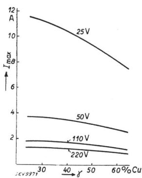
Fig. 6. Grenzstromstärken ( I_{max} ) für Wolfram-Silber-Verbundmetalle in Abhängigkeit von der elektrischen Leitfähigkeit ( \gamma in % \gamma_{Cu} ).
