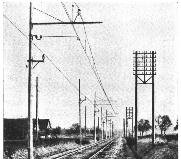
Fig. 8. Parallelführung von Ruten- und Bügefahrlleitung und Schwachstromgestänge.
