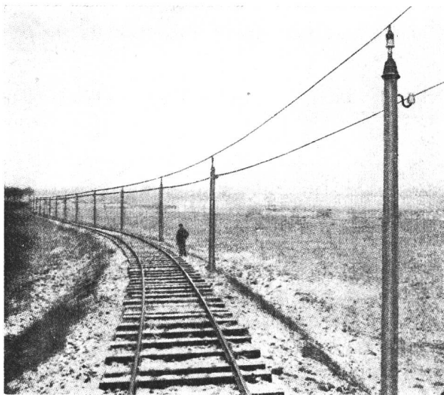
Fig. 7. Rutenfahrleitung auf offener Strecke.
