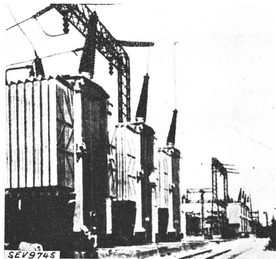
Fig. 6. 287/132-kV-Autotransformatoren. 3 x 80 000 kVA.
