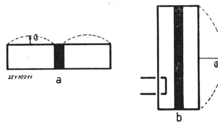
Fig. 3. Hohlraumresonatoren
