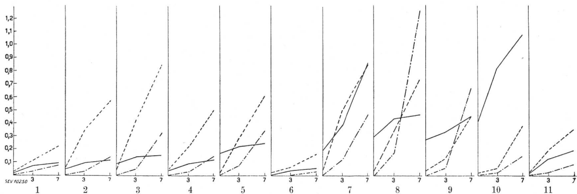
Fig. 1 bis 11. Graphische Darstellung der Resultate der Untersuchung der Oele Nr. 1 bis 11. Abszissen: Prüfdauer (3 und 7 Tage). Ordinaten: - - - - - Säurezahl. - · - · - Schlamm. — Sauerstoffzahl × 0,01.
