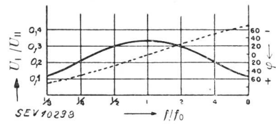
Spannungs- und Phasengang der Schaltung Fig. 18
