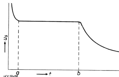
Fig. 9. Elektrische Festigkeit der Oelpapier-Isolation der Transformatoren in Funktion der Beanspruchungsdauer Zwischen «a» und «b» ist die Festigkeit von der Beanspruchungsdauer unabhängig
