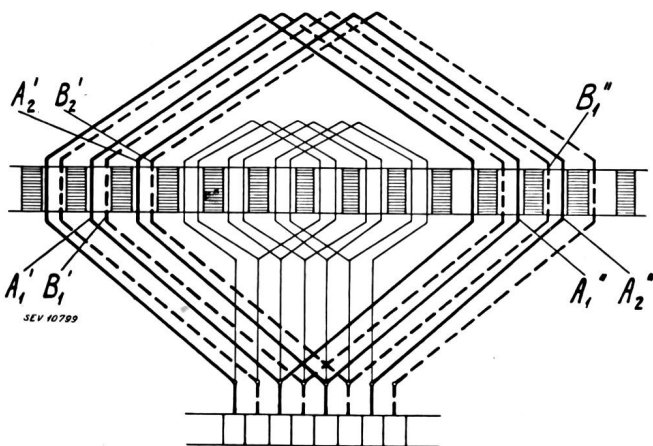
Fig. 16. Zweifachparallelwicklung mit Hilfswicklung mit 2 Lamellen pro Nut. Nutzenzahl pro Pol = 9 y_H = 9 bzw. 10 y_h = 3
