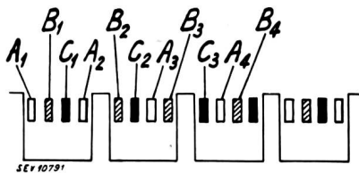
Fig. 12. Dreifachparallelwicklung mit 4 Lamellen pro Nut n = \frac{a}{p} = 3 k = 4
