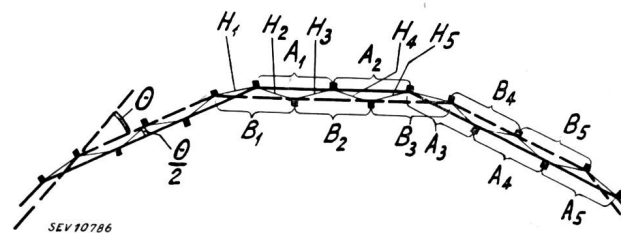
Fig. 8a. Spannungsvektordiagramm der Wicklung nach Fig. 8
