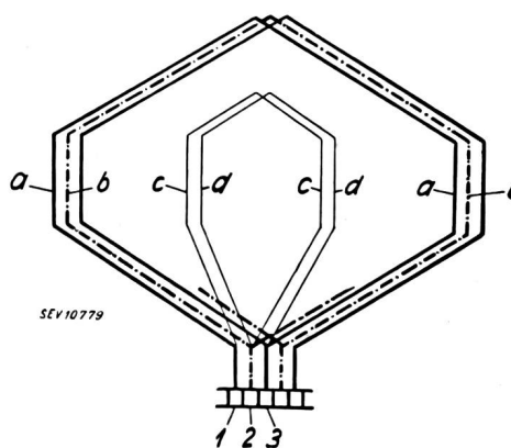
Fig. 3. Zweifachparallelwicklung mit Hilfswicklung nach DRP 660431
