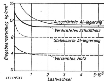
Verschiedene Eigenschaften von verdichtetem Schichtholz
