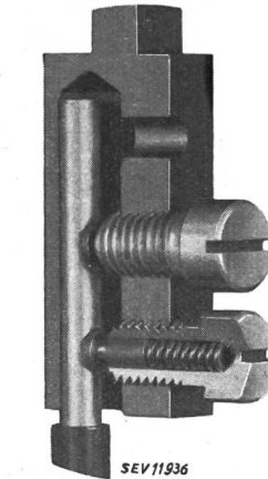
Federnde Druckschraube für Aluminiumdrahtverbindungen (Landis & Gyr)
