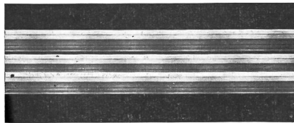
Fig. 27. Drei Leuchtspuren der Argalampe Die Dunkel-Phase der Periode ist pro Streifen fünfmal zu erkennen. Keine Diskontinuität.
