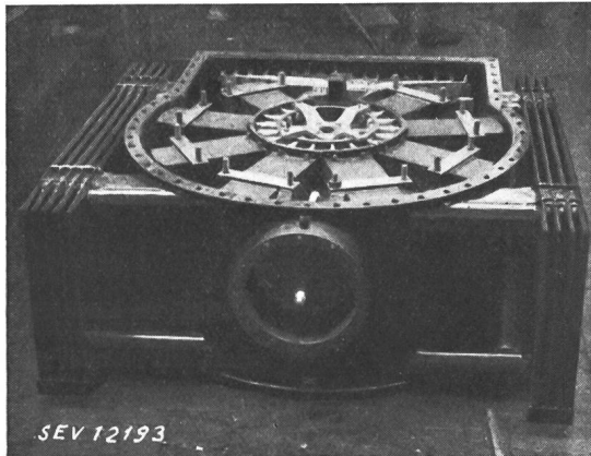
Fig. 14. Triebwagentransformator für 410 kVA, 16 2 / 3 Hz. Flache Bauart für Anbringung unter dem Wagenboden
