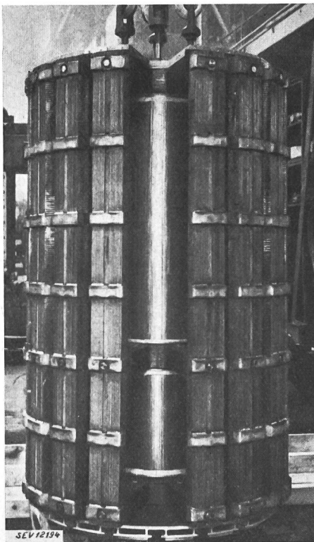
Fig. 15. Eisenkern eines grossen Lokomotivtransformators für 2700 kVA, 16 2 / 3 Hz Radialgeblechter Kern mit quergeblechtem Zwischenjoch, für eine Wicklungsanordnung mit überspannungsseitiger Steuerung
