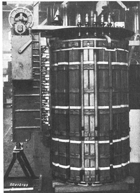
Fig. 16. Aktiver Teil eines grossen Lokomotivtransformators für 2700 kVA, 16 2 / 3 Hz mit angebautem, überspannungsseitigem Stufenschalter
