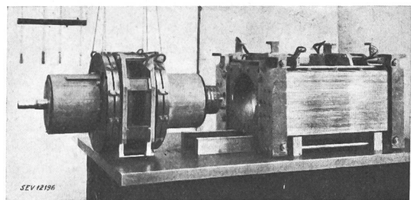
Fig. 17. Telle eines Triebwagentransformators mit radialgeblechtem Drehkern und stufenloser Stromabnahme auf den blanken Sekundärwicklungen
