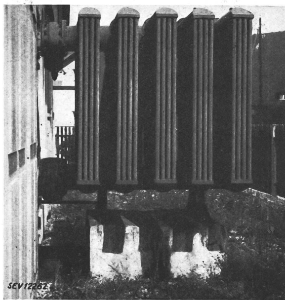
Fig. 4. Kühler der Anlage Fig. 2
