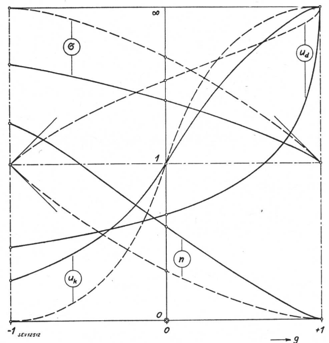
Fig. 3. Scheitelspannungskorrekturfaktor \sigma und Differenzspannungswert u_d
