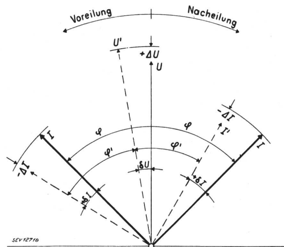
Fig. 1. Wirkung der Messwandlerfehler U, I, \varphi, P Sollwerte, wobei P = U I \cos \varphi U', I', \varphi', P' Istwerte P' = U' I' \cos \varphi' Gesamte Messfehler in % bei einer Einphasenmessung: bei Nacheilung \approx \Delta U \% + \Delta I \% - 0,0291 (\delta U - \delta I) \operatorname{tg} \varphi bei Voreilung \approx \Delta U \% + \Delta I \% + 0,0291 (\delta U - \delta I) \operatorname{tg} \varphi Sämtliche Einzelfehler sind einschliesslich ihres Vorzeichens einzusetzen, wobei \delta_{\text{vor}} = +, \delta_{\text{nach}} = - gilt.
