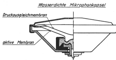
Fig. 5a. Wasserdichte Mikrophonkapsel (Uster)
