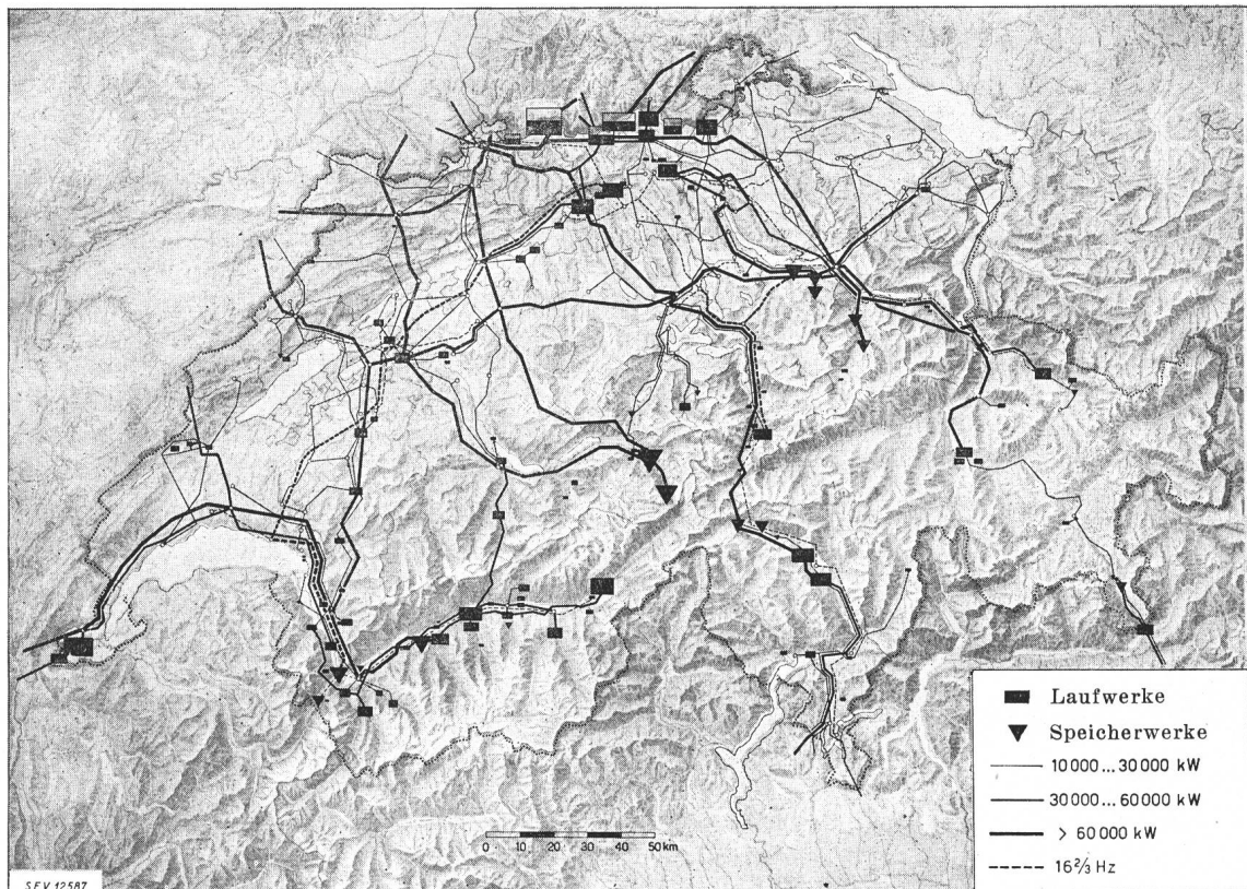
Fig. 6. Situationsplan der Schweiz. Elektrizitätswerke von mehr als 1000 kW Leistung und der Hauptübertragungsleitungen 1945 1 : 2 500 000
