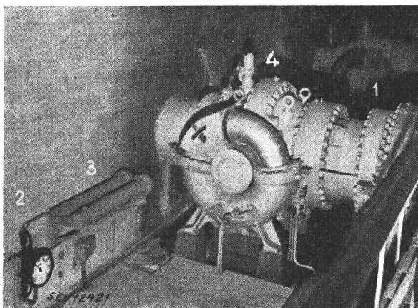
Fig. 13. Venturi-Wassermesseinrichtung in der Schieberkammer des Kraftwerkes Innertkirchen
