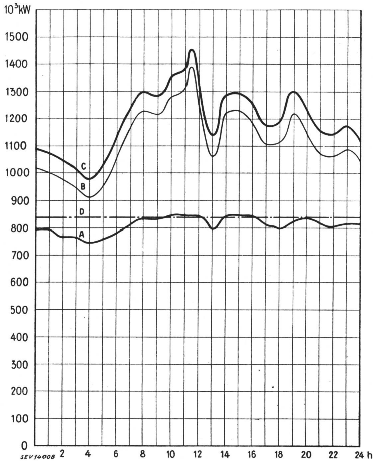
Tagesdiagramme der beanspruchten Leistungen, Mittwoch, den 18. September 1946
