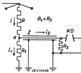
Fig. 14. Verzögerungskabel mit Widerstandsabschluss an beiden Enden
