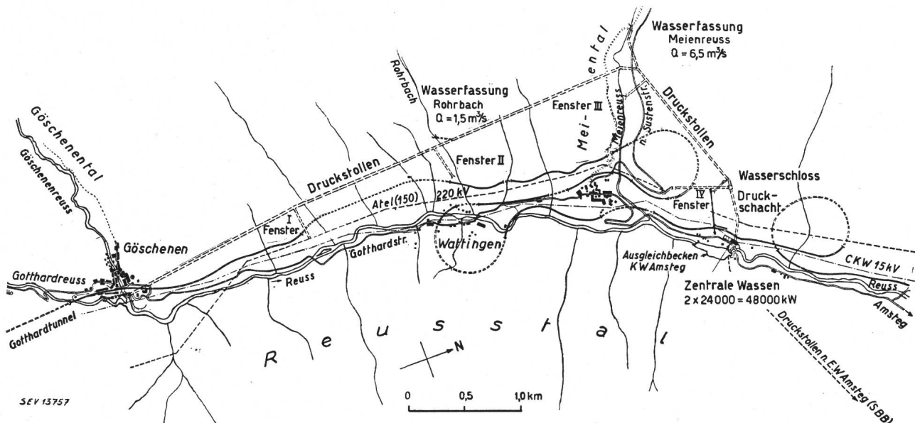
Fig. 1. Kraftwerk Wassen, Ubersichtsplan
