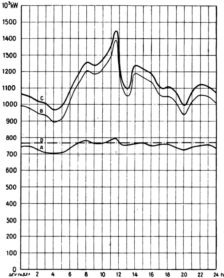
Tagesdiagramme der beanspruchten Leistungen, Mittwoch, den 18. Juni 1947
