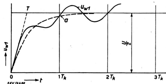
Fig. 5 Zeitlicher Verlauf der Windungsspannung der ersten Windung (für den Fall T/T k = 1/2) Bezeichnungen wie in Fig. 4
