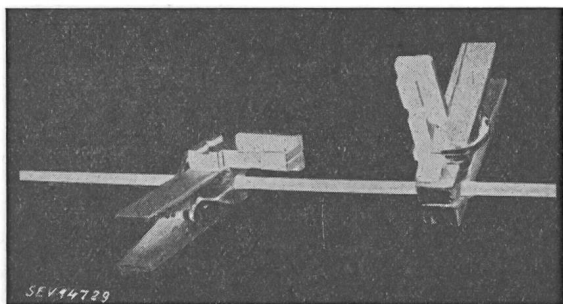
Fig. 8 Stahlstäbchen in Kunstharzfassung auf Telephon- oder Niederspannungsleitung aufgesetzt
