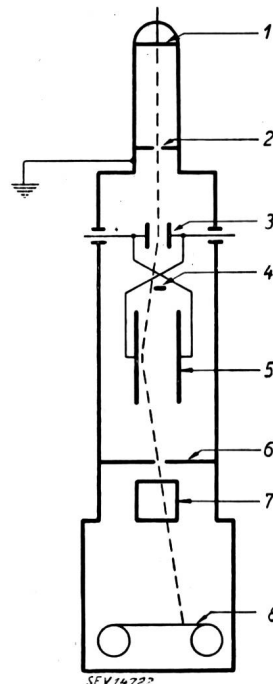
Fig. 1 Vom Verfasser entwickelte Schaltung des Kathodenstrahl-Oszillographen für 40 kV Gleichspannung 1 Kathode 2 Anodenöffnung 3 Ablenkplatten 4 Sperrelektrode 5 Ablenkplatten 6 Schirmplatte 7 Zeitkreisplatte 8 Film
