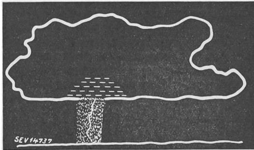
Fig. 16 Einleitende Entwicklung eines Blitzes von einer negativ geladenen Wolke zur Erde
