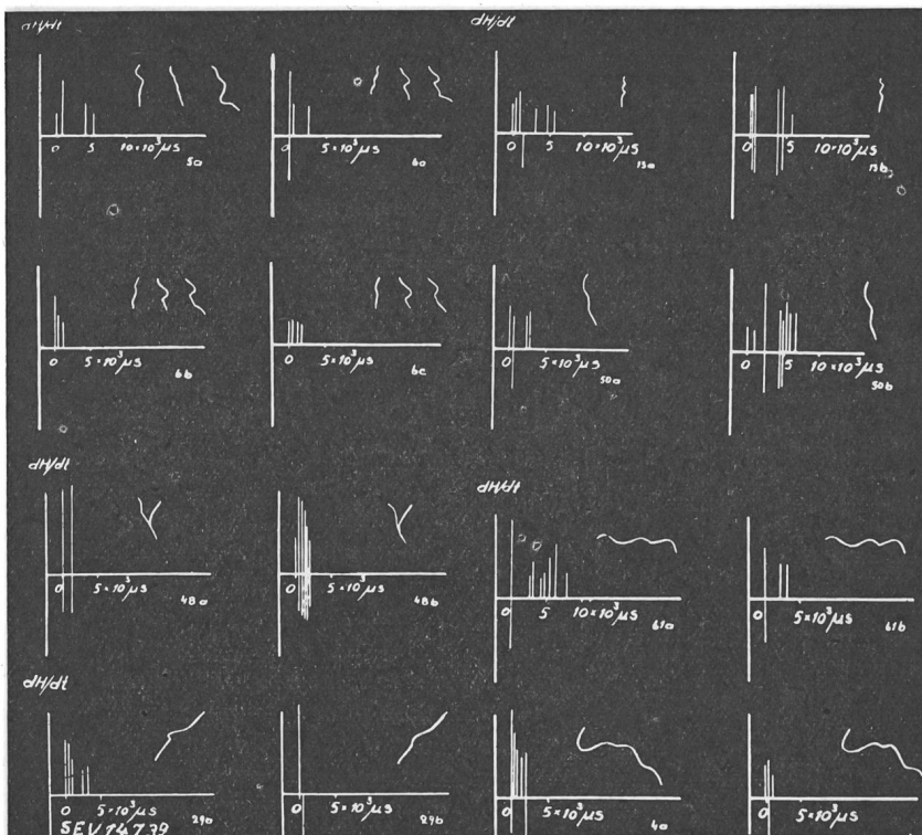
Fig. 19 Variationen des magnetischen Feldes von Mehrfachblitzen im gleichen Blitzkanal
