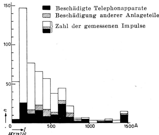
Fig. 9 Störströme in A auf schwedischen Telephonleitungen im Jahre 1943
