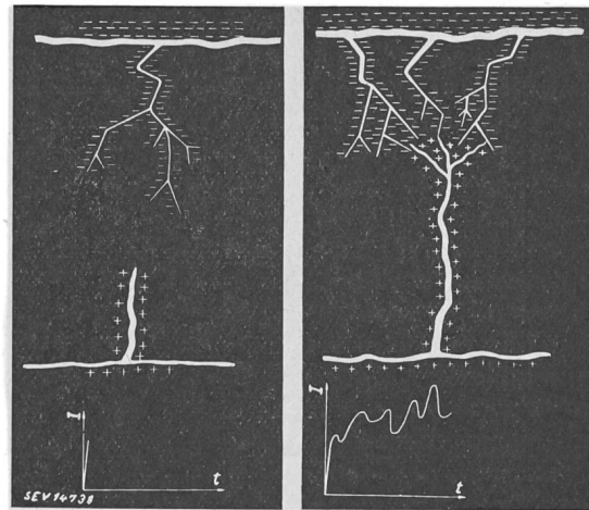
Fig. 17 Beginn der Hauptentladung eines Blitzes aus einer negativ geladenen Wolke zur Erde
