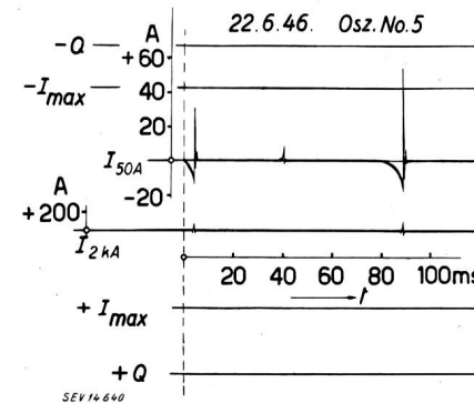
Fig. 10 Wirkung eines dem Blitzableiter benachbarten Blitzeinschlages
