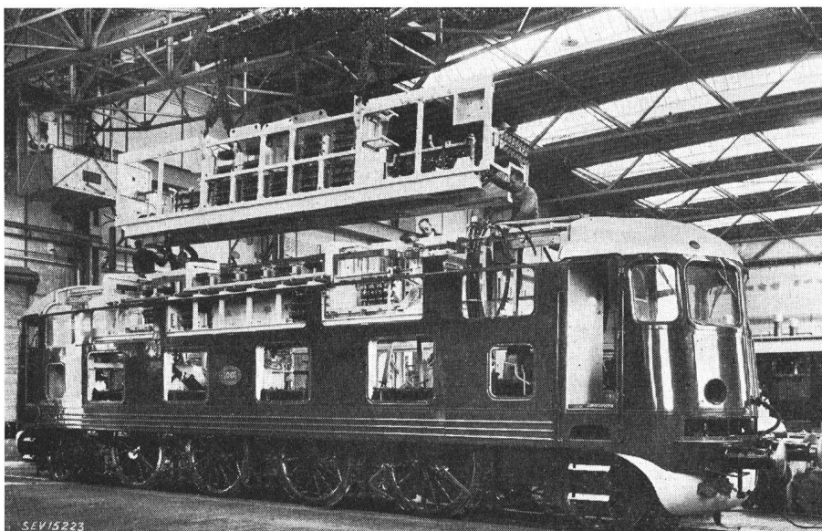
Fig. 2 Die Lokomotive während der Montage Oben ist das Eisengerüst für die elektrischen Apparate herausgehoben. Lücken im Lokomotivkasten dienen zum Einschleiben der Triebmotoren
