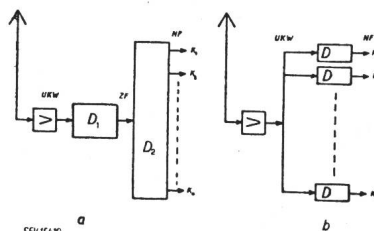
Fig. 6 Empfänger a Einträgersystem; b Mehrträgersystem; D, D_1, D_2 Demodulatoren; K_1, \dots, K_n niederfrequente Nachrichtenkanäle
