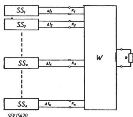
Fig. 7 Verwendung einer Frequenzweiche SS1...n Sendesysteme; \Delta f_{1...n} zugehörige Frequenzbänder; K1...n Eingangsklemmen; W Frequenzweiche; R Belastungswiderstand
