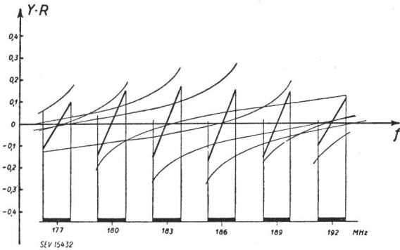
Fig. 19 Totale Eingangsreaktanz
