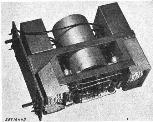
Fig. 7 Zweistufiges Kristallfilter
