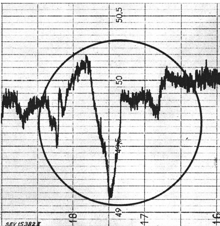
Fig. 17b Frequenz am 10. Juni 1948
