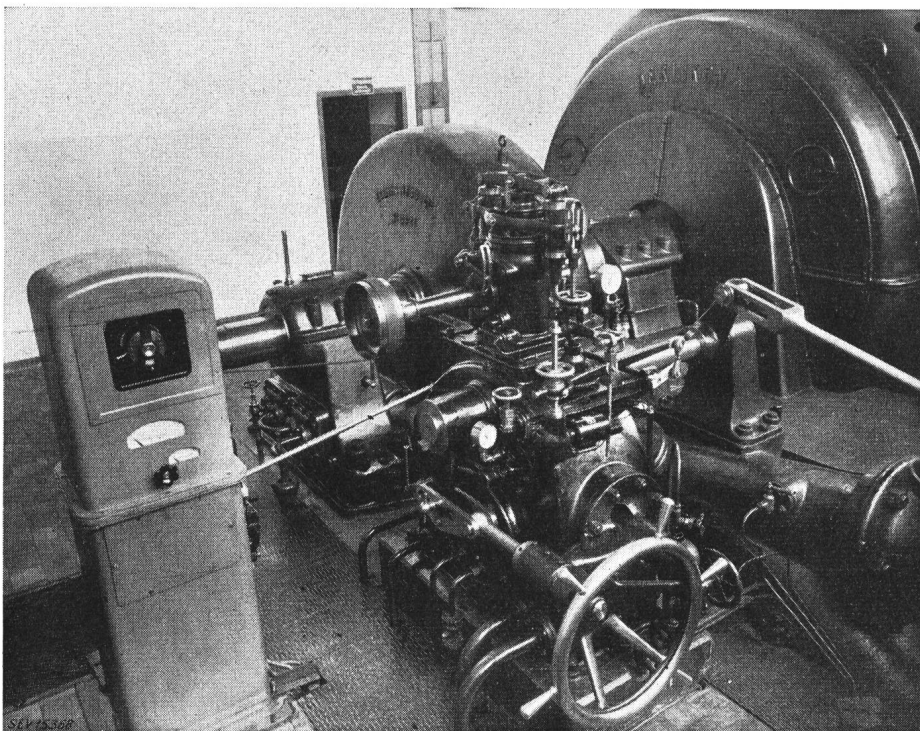
Fig. 4 Erster Versuchs-Leistungsregler Schwanden
