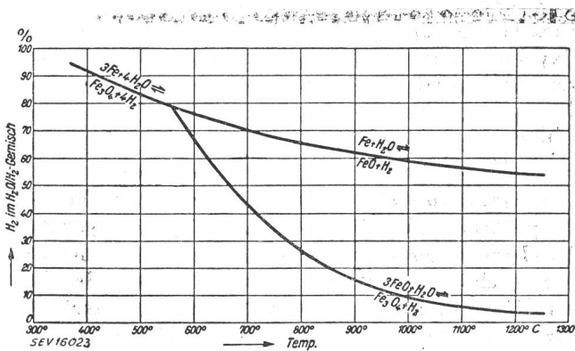
Fig. 7 Gleichgewichte von Wasserstoff-Wasserdampf-Gemischen über Eisen und Eisenoxyden
