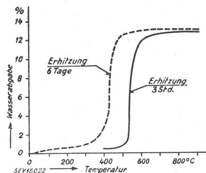
Fig. 6 Wasserabgabe bei bei verschieden langer Erhitzung von Kaolin
