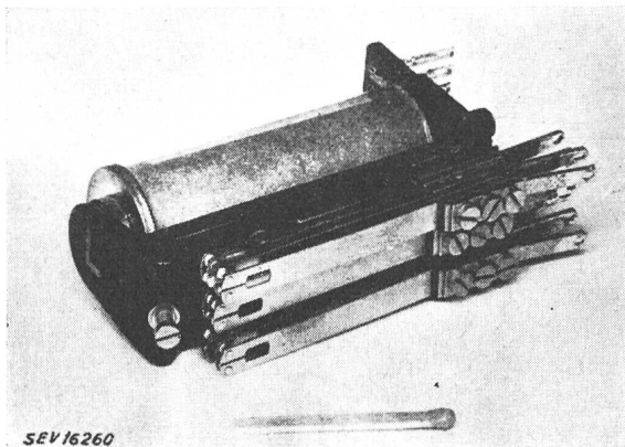
Fig. 8 Relais-Federsatz
