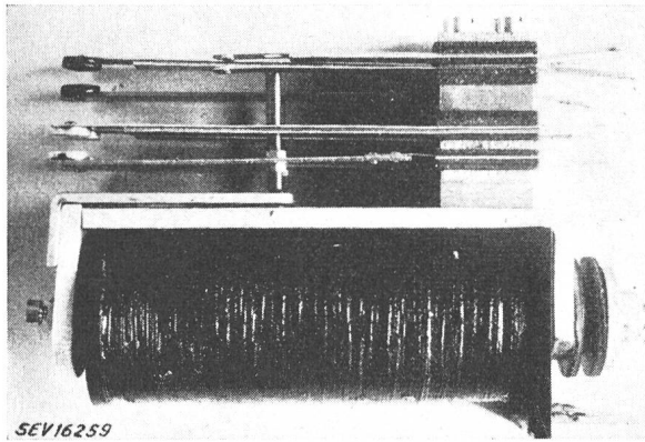
Fig. 7 Relais-Federsatz mit Zwischenlage aus Hartpapier
