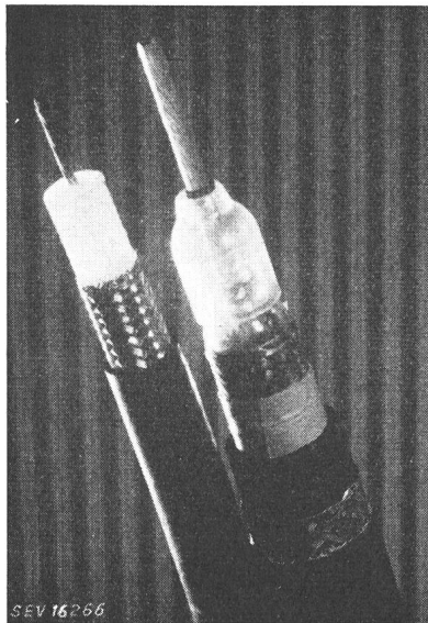
Fig. 14 Hochfrequenzkabel rechts: mit Polystyrolperlen links: mit Polythen- Vollisolation
