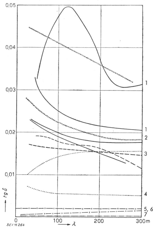
Fig. 12 Verlustfaktor tg δ einiger Isolierstoffe in Funktion der Wellenlänge λ des Prüfstromes 1 Hartpapiere 5 Mycalex 2 Kunstharzpreßstoffe 6 Steatit (Rastea) 3 Kondensatorenpapier roh 7 Glimmer 4 Porzellan
