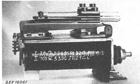
Fig. 9 Relais-Federsatz
