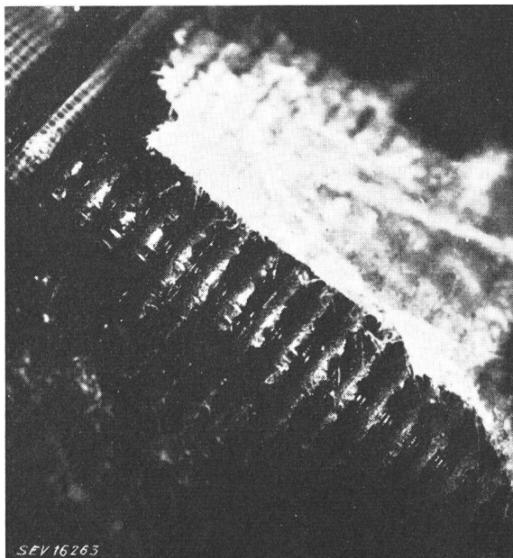
Fig. 11 Korrodiertes Spulenkörper
