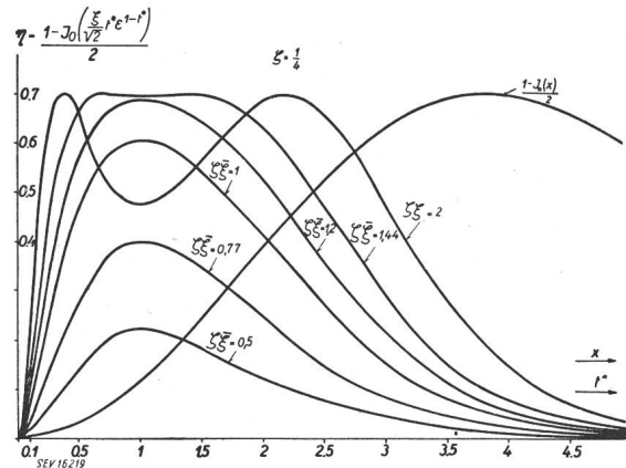
Fig. 9 Aufhellungskurven in Funktion der Zeit für ein Bildelement
