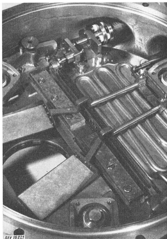
Fig. 11 Wechselkassette
