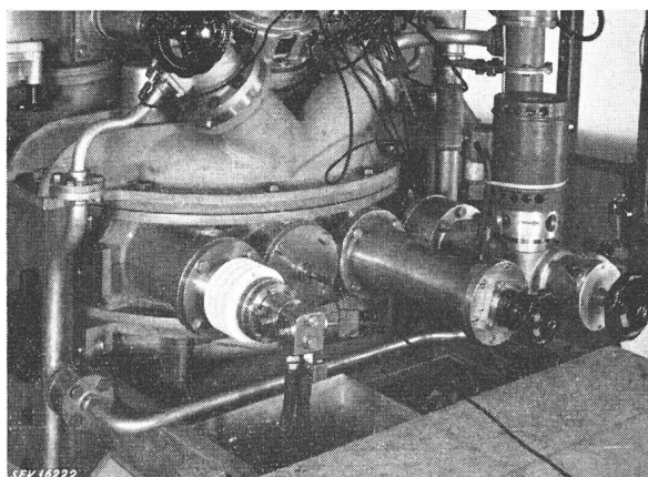
Fig. 12 Kassette eingebaut
