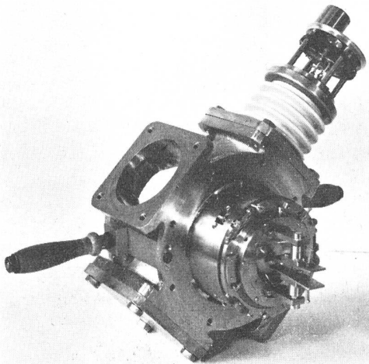
Fig. 22 Kathodenstrahlrohr
