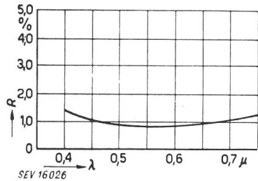
Fig. 3 Experimentelles Reflexionsvermögen einer Einfachschicht aus Kryolith \lambda Wellenlänge; R Reflexionsvermögen
