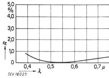
Fig. 2 Theoretisches Reflexionsvermögen einer Einfachschicht \lambda Wellenlänge; R Reflexionsvermögen
