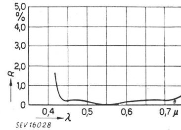
Fig. 2 Theoretisches Reflexionsvermögen einer Einfachschicht \lambda Wellenlänge; R Reflexionsvermögen
