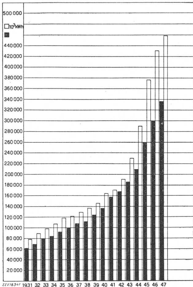
Fig. 1 Haushaltkochherde schwarz: Zahl der Apparate; weiss: Verbrauch
