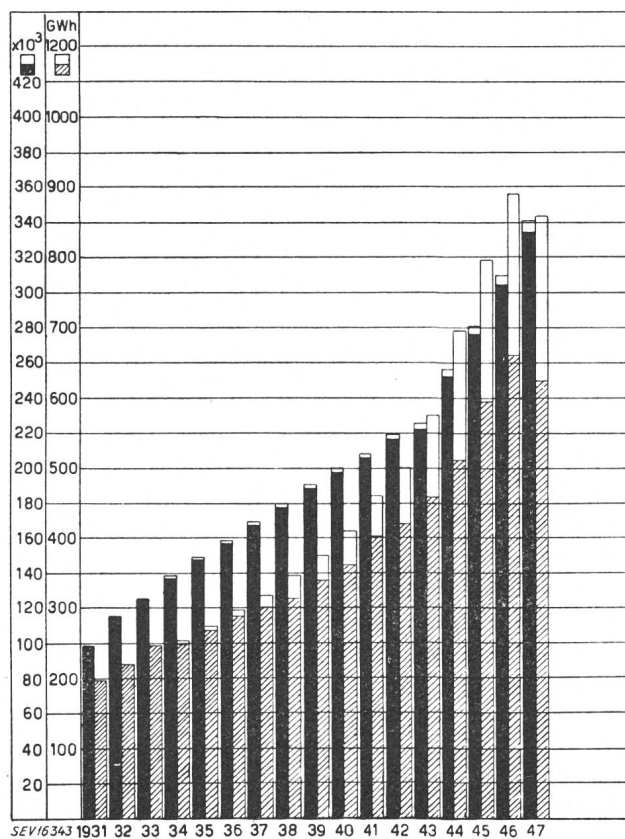
Fig. 3 Heisswasserspeicher und Futterkochkessel schwarz: Zahl der Apparate; schraffiert: Verbrauch; weiss: Anteile für Grossheisswasserspeicher (bis 1943 geschätzt)
