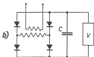
Schaltungen für Vollweggleichrichter a) mit 2 Pufferdrosseln D/2 ; b) mit Pufferkondensator C ; c) mit 2 Pufferkondensatoren 2C in Spannungsverdopplungs-Schaltung nach Greinacher
