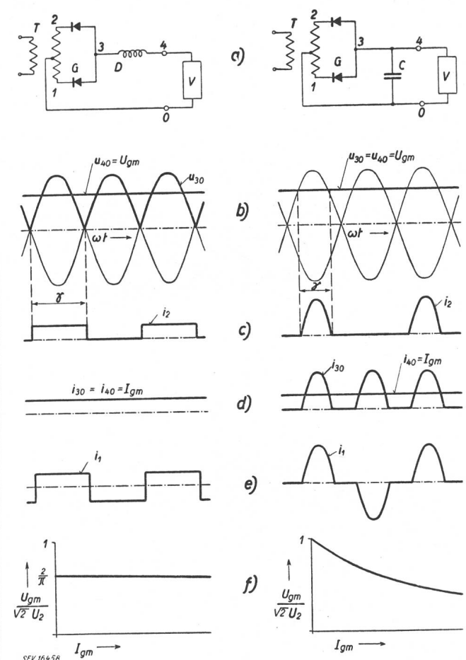
Fig. 1 Gegenüberstellung der zweiphasigen Einweggleichrichterschaltungen mit Pufferdrossel (links) und mit Pufferkondensator (rechts) a) Schaltbilder: T Transformator (sekundär zweiphasig); G Gleichrichterstrecke; D Pufferdrossel; C Pufferkondensator; V Verbraucher; 0...4 Potentialpunkte b) Verlauf der Gleichrichterspannungen u_{30} und u_{40} . U_{gm} erzeugte Gleichspannung (arithmetischer Mittelwert); \omega Kreisfrequenz; t Zeit c) Verlauf des Sekundärstroms i_2 durch eine Gleichrichterstrecke \gamma Brenndauer der Gleichrichterstrecke d) Verlauf der Gleichrichterströme i_{30} und i_{40} und des Gleichstromes I_{gm} (arithmetischer Mittelwert) e) Verlauf des Primärstromes i_1 des Transformators f) Belastungskennlinien: U_2 Sekundärspannung der einzelnen Gleichrichterstrecke; U_{gm} Gleichspannung; I_{gm} Gleichstrom (Belastung)
