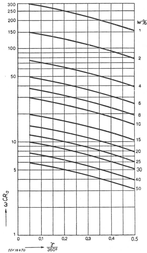
Fig. 12 Diagramm zur Berechnung von Gleichrichterschaltungen C Kapazität des Pufferkondensators; R_a Aussenwiderstand; w Welligkeit; \gamma Brennweite
