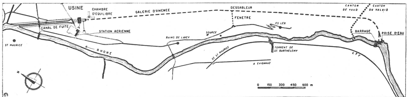
Fig. 20 Lavey Plan de situation
