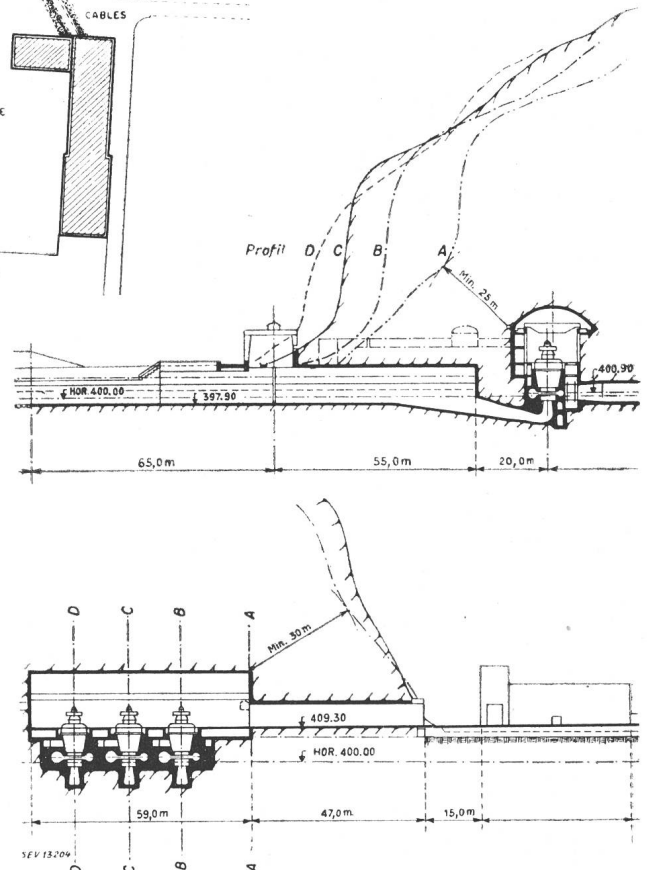
Fig. 25 Lavey Usine souterraine, coupes
