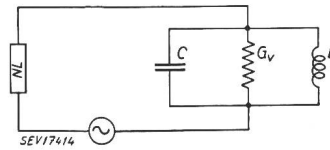
Fig. 6 Schwingkreis mit äusserer Wechselspannung
