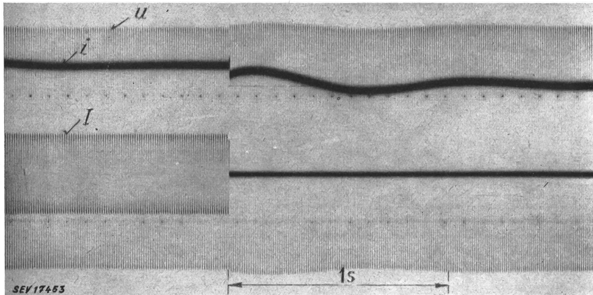
Fig. 8 Relevé du comportement du générateur à la suite d'une brusque variation de la charge u = Tension du générateur i = Courant d'excitation I = Courant de charge
